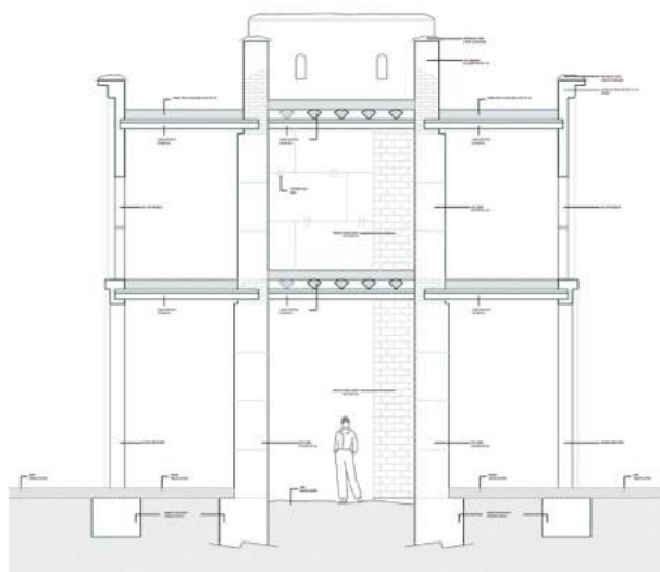
Figura 6: Estudio tipológico y constructivo de la qasbah tradicional.
